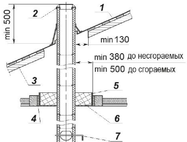
Рисунок 3. Схема дымовой трубы.
