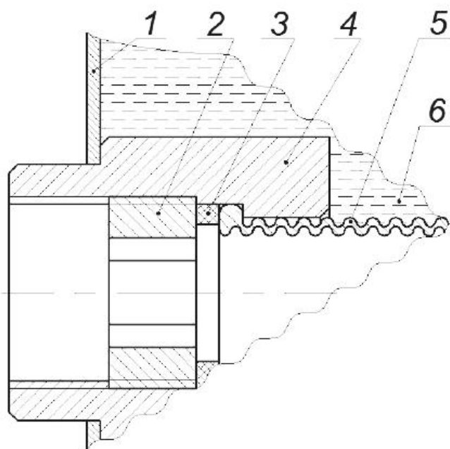
Рисунок 7. Резьбовой фитинг проточного водонагревателя.
