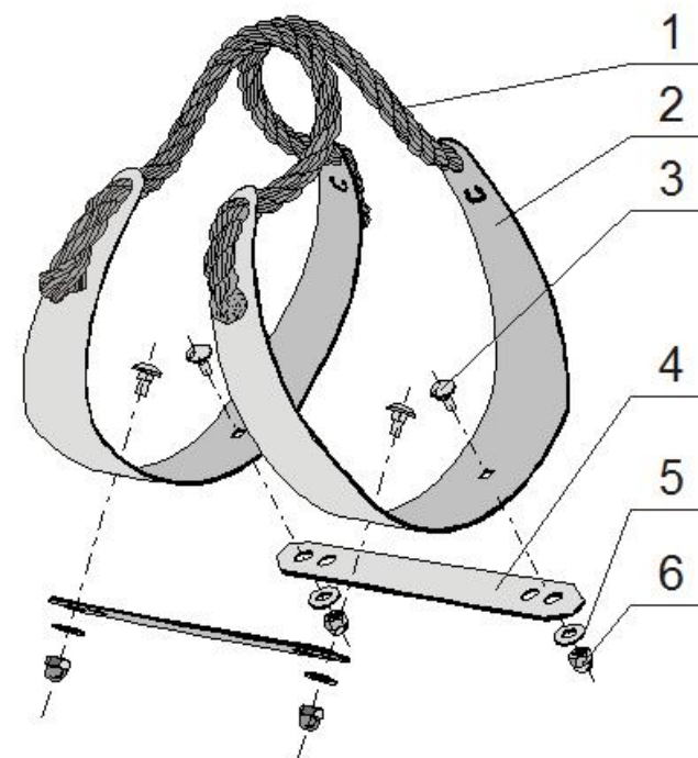
Рисунок 1. Сборка дровницы
