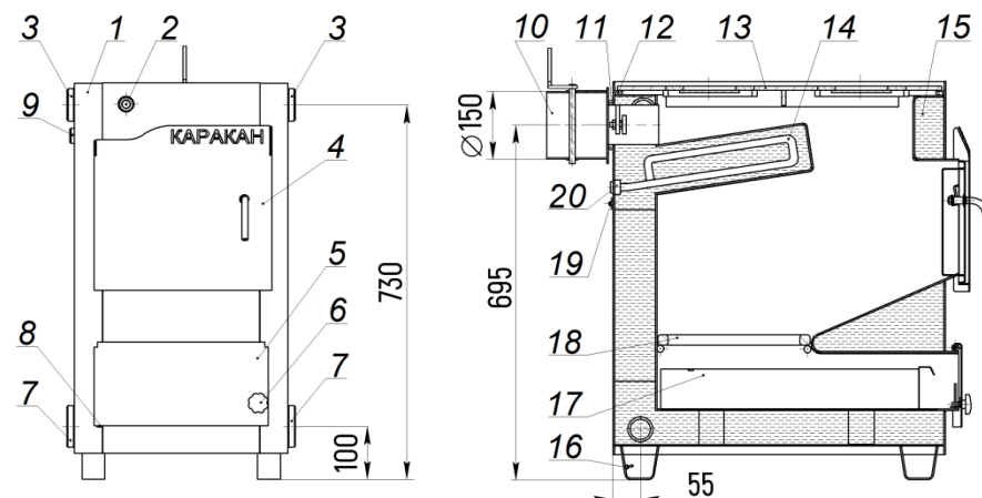
Рисунок 1. Устройство котла. Базовая комплектация
