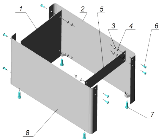
Рисунок 1. Сборка корпуса подставки.
