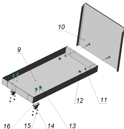
Рисунок 2. Сборка выкатного поддона.
