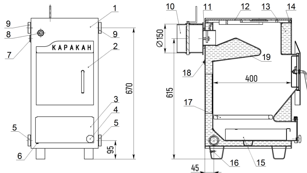
Рисунок 1. Схема котла. Базовая комплектация
