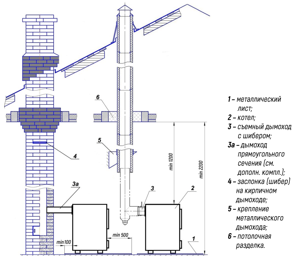
Рисунок 2. Схема монтажа котла и дымовой трубы
